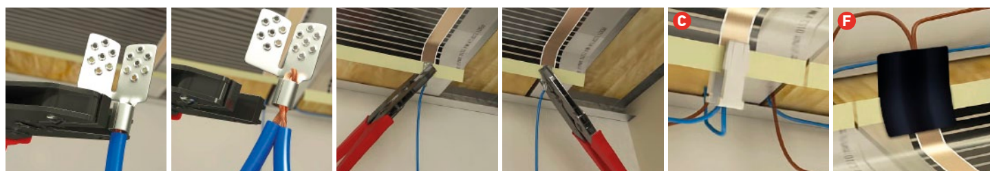
C ECOFILM C – Installierung des Steckverbindingengehäuses; F ECOFILM F – Verbinding parallel zum Mastix
